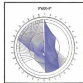
Poti potresnih valov skozi notranjost Zemlje.
